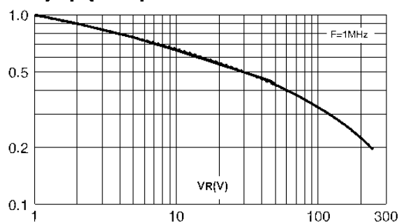
C_o 随偏置电压的变化率 (相对于 V_R=1V )
